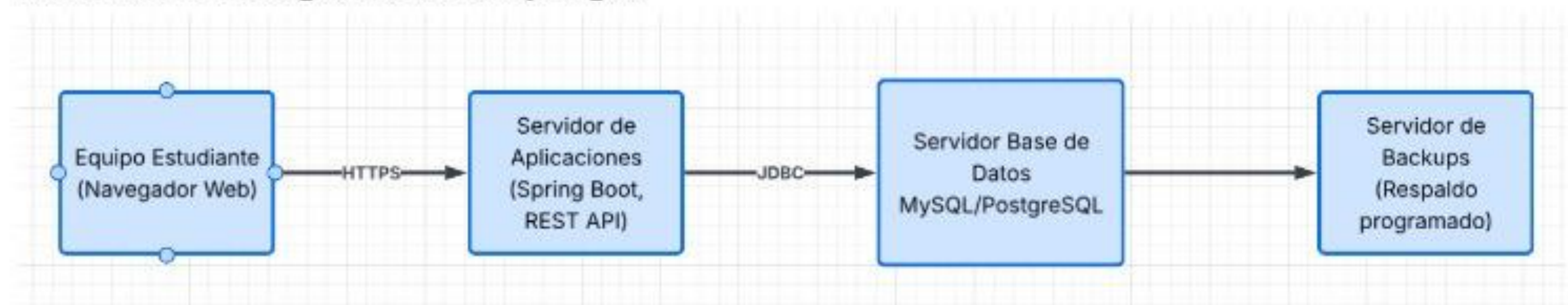
Ilustración 6: Diagrama de Despliegue
