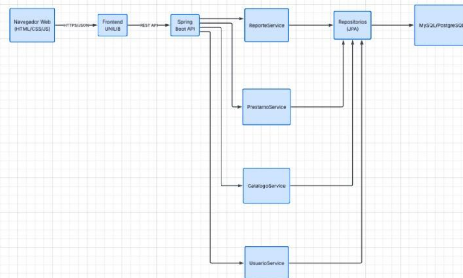
Ilustración 2: Diagrama de Componentes y Conectores
